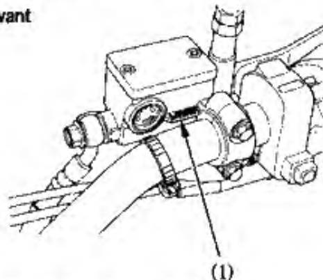
(1) Repère de niveau inférieur (LOWER)
