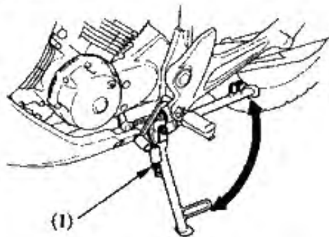
(1) Ressort de la béquille latérale
